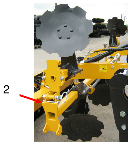
Figure 5 : Disque de bordure replié
